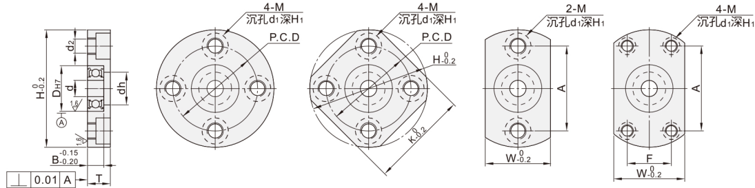
圆法兰
