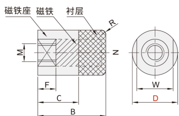
内螺纹型 YLQ21
