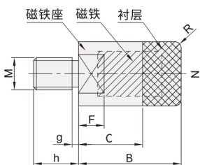
外螺纹型 YLQ11/12
