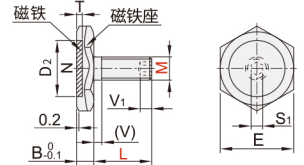
超薄短头内六角孔型 YLL46
