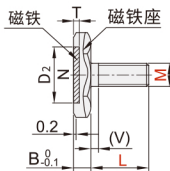
超薄短头型 YLL41
