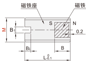
一字槽型 YLK21/22
