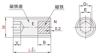
内六角孔型 YLK31/32
