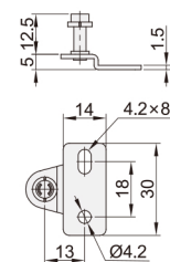
标配件B
