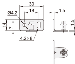
标配件A
