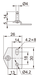
标配件B
