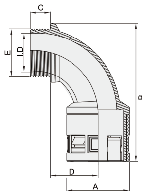
DQA75 软管直角接头
