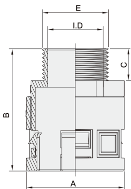
DQA74 软管金属螺纹接头
