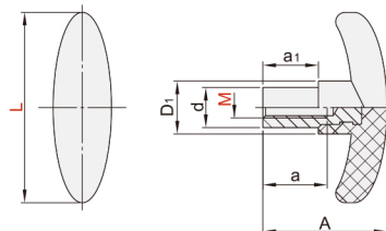
T型把手 STA21
