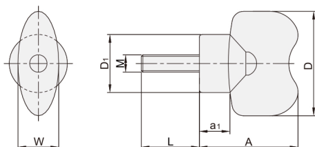
外螺纹型 STA31
