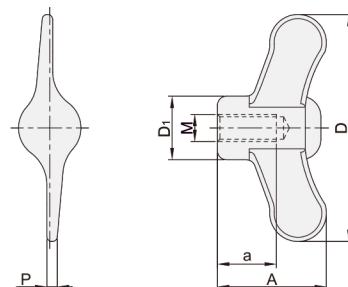
内螺纹型 STA41
