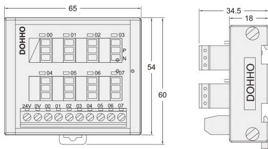
MTM081/MTM081-P
