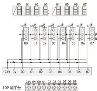
MTM081
