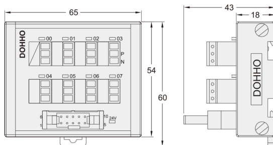
MTM080/MTM080-P
