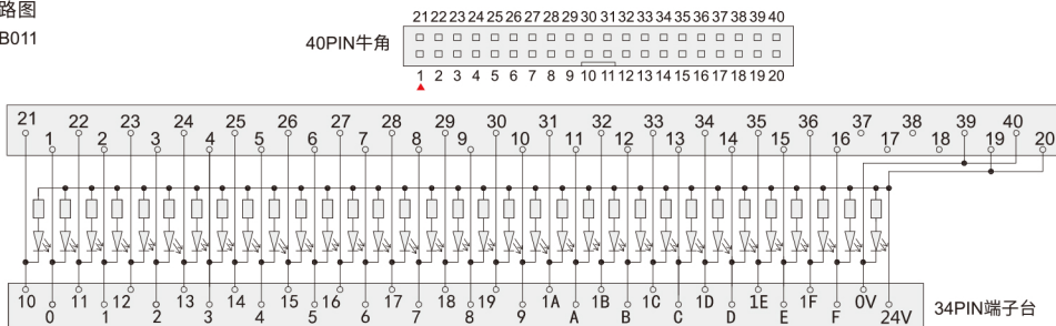
电路图
