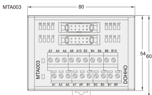
外形图
