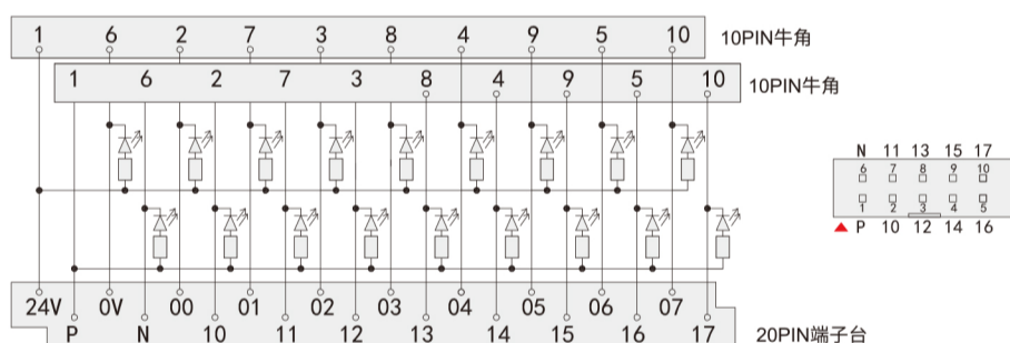
电路图 MTA003
