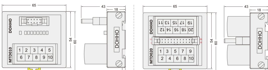
外形图 MTD010
