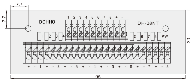
外形图 DH-08NT1
