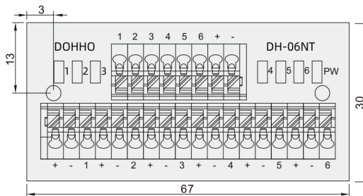
外形图 DH-06NT1
