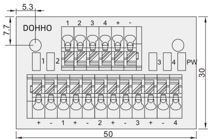
外形图 DH-04NT1
