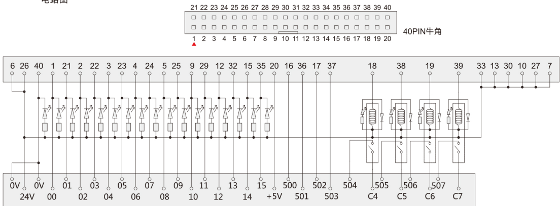
电路图
