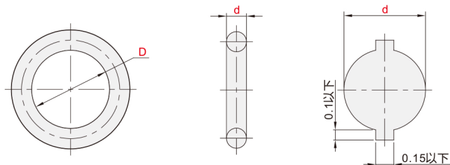
截面放大图
