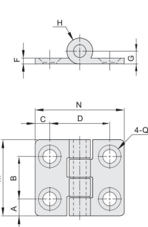
短型 VKT01/VKT02
