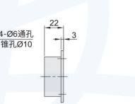
开孔尺寸
