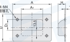
开孔尺寸
