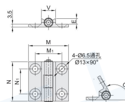
锥孔型 VKC31
