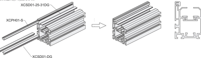
钢轨型材(DG)使用示例
