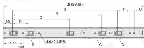
外轨安装孔位图
