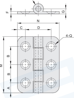
加长型 VKV01/VKV02
