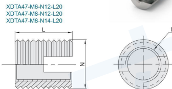
视图标准：第三视角
