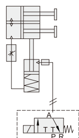
气路图:
