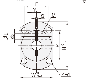
对边法兰型ZPM11/12/16
