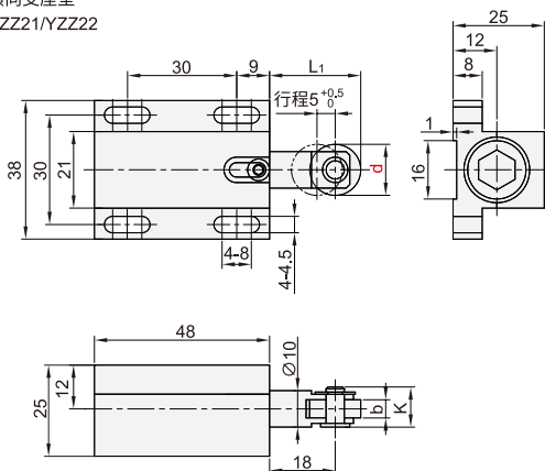
横向支座型 YZZ21/YZZ22
