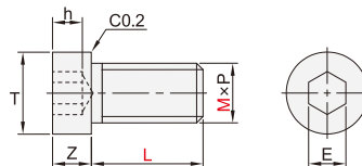
短头小径内六角圆柱头螺钉 YWP13/14
