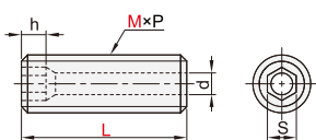
内六角紧定螺钉型 YWK45
