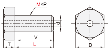
六角头型 YWK44
