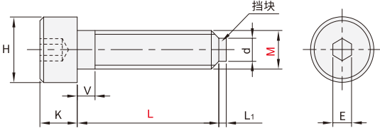
直杆型 YTC01/02/11/12
