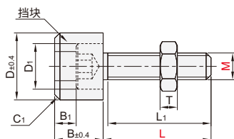
内六角圆柱挡块 YTC31/32/51/52
