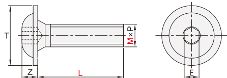
内六角平头带垫螺钉 YWD06/07
