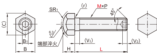
圆头内六角孔型
