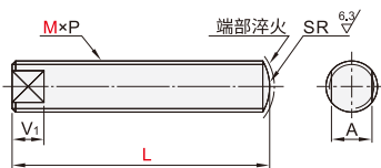
带扳手槽型
