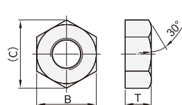
■螺帽尺寸
