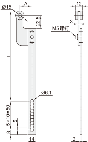
带眼多孔连杆 XAG51
