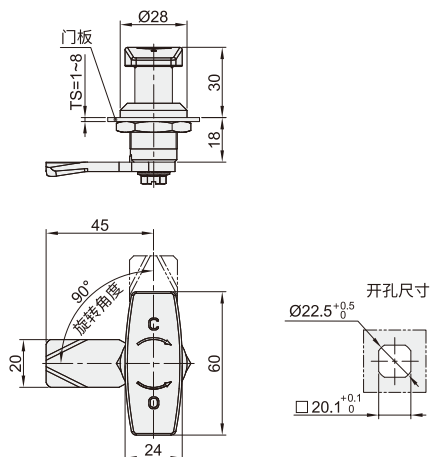
60系列-无锁芯 XAB54
