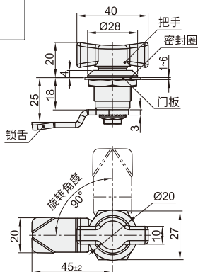
止口高度 25 无锁芯 XAB47
