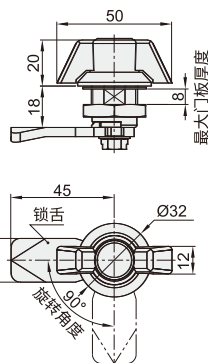
止口高度: 18 无锁芯 XAB49
