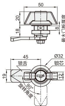
止口高度: 18 一字形锁芯 XAB48
