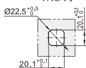
开孔尺寸
