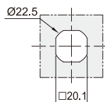
开孔尺寸
