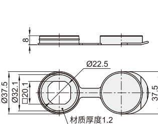
防尘盖
