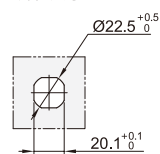
■开孔尺寸
