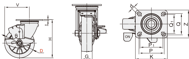
五金双刹 WHB03
