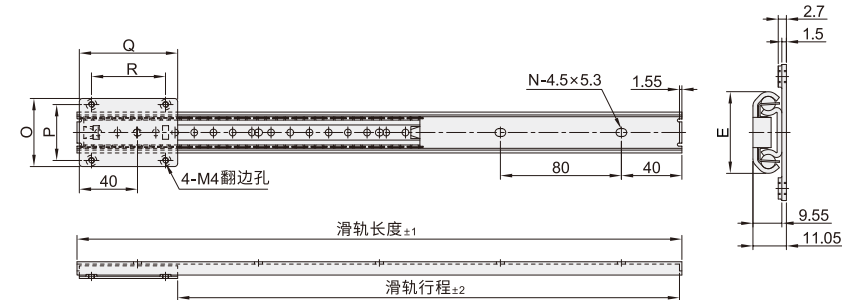
螺纹孔型 VZS01
