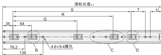
外轨安装孔位图
