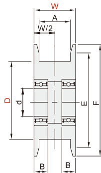
带法兰 双轴承
