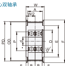
中心双轴承
