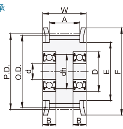
双轴承
