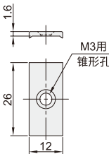
吸附板
