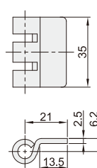
活动连接件
