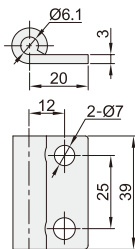
活动连接件
