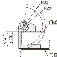
安装图
