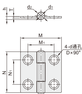
锥孔型 VKJ05
