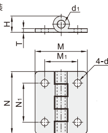
4孔安装
