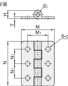
6孔安装
