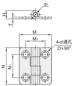
VKH11 4孔安装
