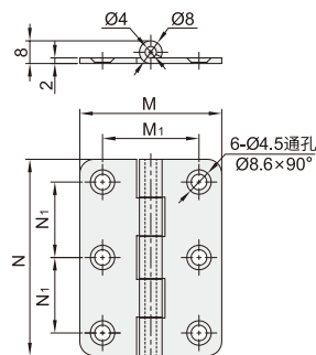
VKH16 6孔安装
