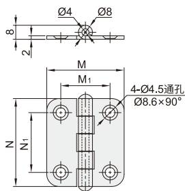
VKH16 4孔安装
