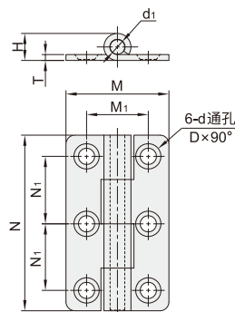
VKH11 6孔安装
