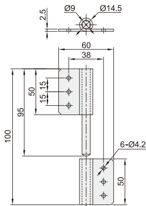
圆孔型 VKF41/42
