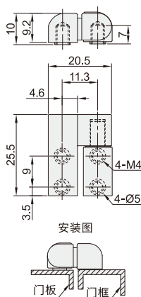
对称型 VKF25/26 规格: 2620
