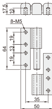
对称型 VKF25/26 规格: 2620A
