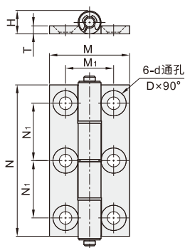
经济型 6孔安装
