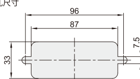
开孔尺寸
