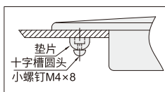
安装图
