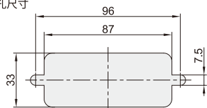
开孔尺寸
