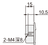
安装图
