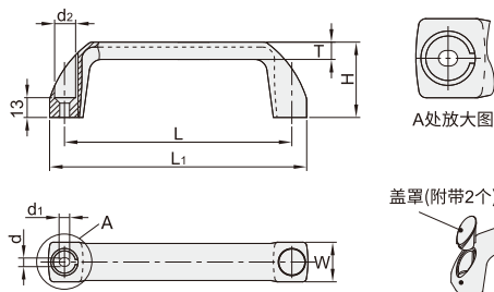
圆角带盖型 VFT71
