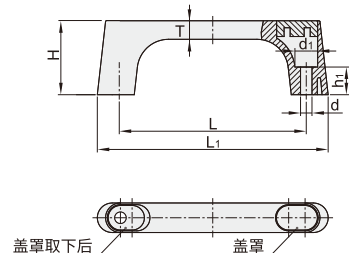
斜角带盖型 VFT76
