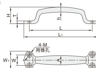
弧型 VFE15 用途：车辆、室内外的大型门。
