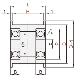
H=16·21·27·32
