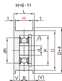
法兰型 VBG01/02/04/11
