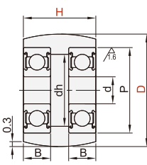
H=16·21·27·32
