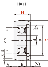
圆弧型 VBG21/22/24/31/36
