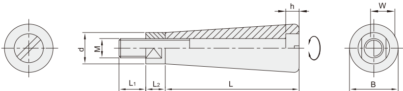
SUG61 外螺纹式
